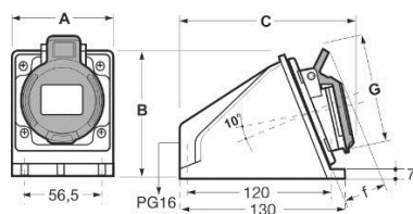
Montaje bases de 16A / 16A socket mounting
