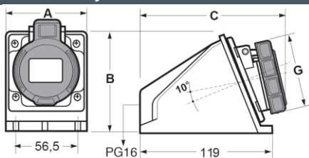
Montaje bases de 16A / 16A socket mounting
