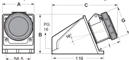
Montaje bases de 32A / 32A socket mounting
